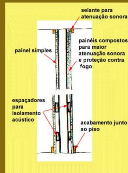
corte esquemático
